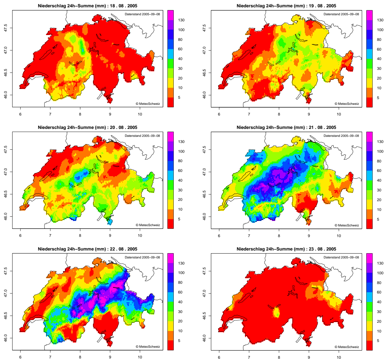
Figur 2: Niederschlagsverlauf vom 18.-23. Aug. Die Analysen zeigen die 24 Stunden Summe jeweils von 8 Uhr bis 8 Uhr (MESZ) des Folgetages. Die Farbskala unterscheidet sich von jener in Figur 1. In den beiden Tagen vor dem Hauptereignis (19./20. August) ist über weite Gebiete des Landes bereits intensiver Regen gefallen. Im Verlaufe des Ereignisses hat sich die Niederschlagsaktivität von den Voralpen ins Innere der Alpen und gegen Osten verlagert.
