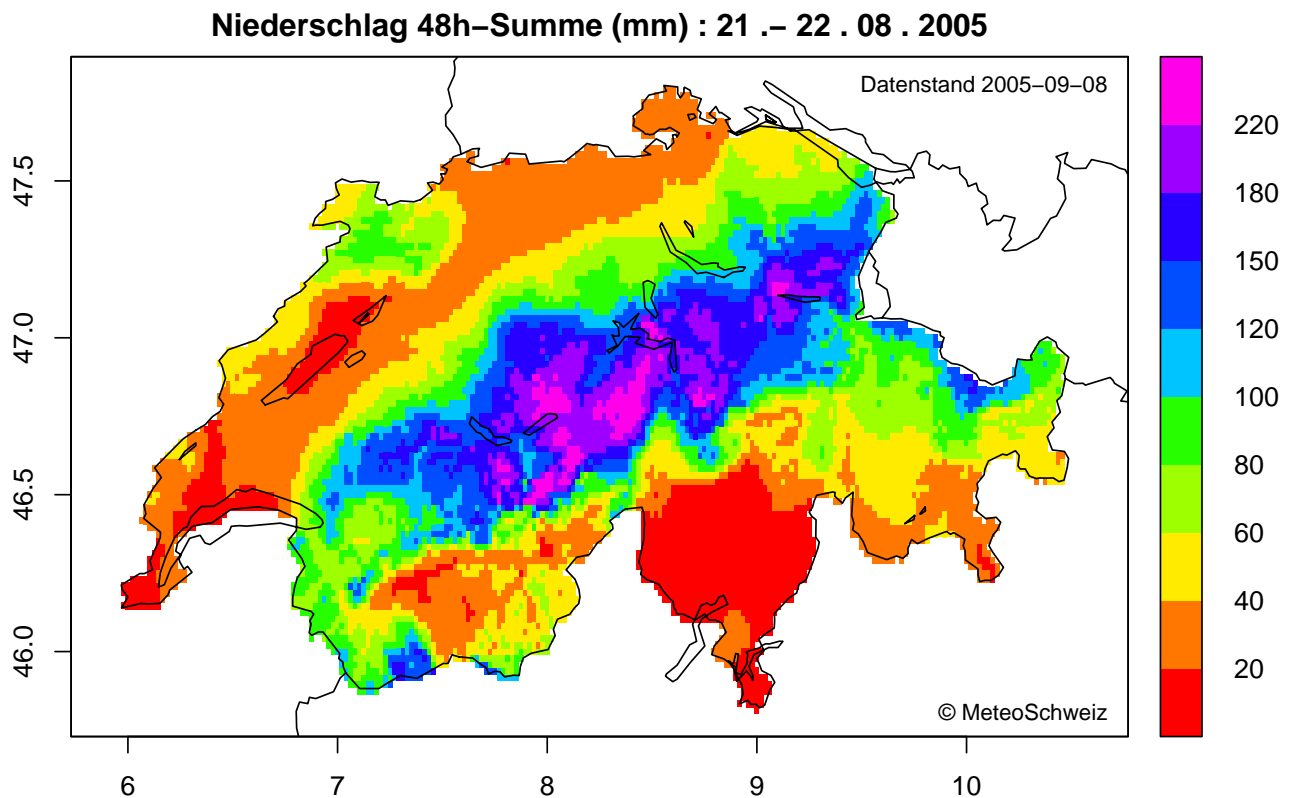
Figur 1: Niederschlagssumme (in l/m^2 ) für die zwei Tage Sonntag / Montag 21./22. August 2005. (Exakte Periode: 21.8. 8:00 MESZ bis 23.8. 8:00 MESZ). Die Analyse wurde aus Messungen an 372 Stationen der MeteoSchweiz (konventionelle, automatische und Niederschlagsstationen) und 42 IMIS-Stationen des SLF gerechnet (Datenstand 8.9.05). Einzelne Stationen haben bis zu 300 l/m^2 gemessen.
