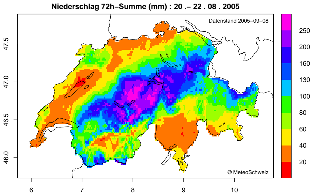
Figur 3: Analog zu Figur 1 aber für die drei Tage Samstag bis Montag 20.-22. August 2005. (Exakte Periode: 20.8. 8:00 bis 23.8. 8:00 MESZ). Die Farbskala unterscheidet sich von jener in Figur 1.
