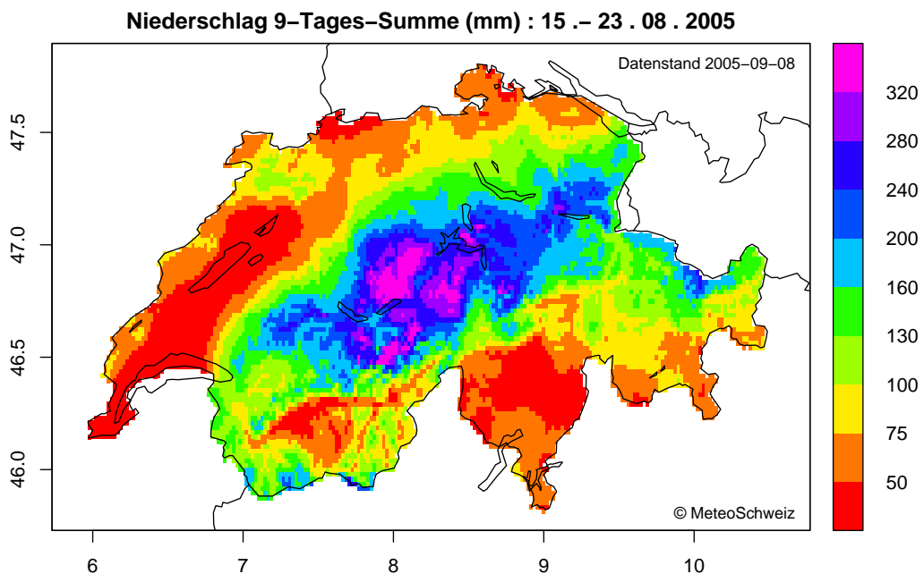
Figur 4: Analog zu Figur 1 aber für die 9 Tage 15.-23. August 2005. (Exakte Periode: 15.8. 8:00 bis 24.8. 8:00 MESZ). Die Farbskala unterscheidet sich von jener in Figur 1.
