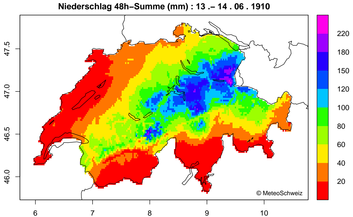
Figur 6: Niederschlagsverteilung für die 2 Tage 13.-14. Juni 1910. Damals hat eine ähnliche Wetterlage zu schweren Regenfällen und Hochwassern geführt. (Zu vergleichen mit Figur 1.) Die Niederschlagsanalyse für dieses Ereignis beruht auf Beobachtungen an nur 104 Messstationen und ist deshalb nur bedingt mit Figur 1 vergleichbar.
