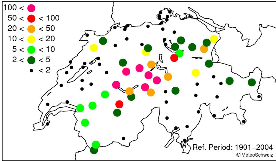
Figur 5: Geschätzte Wiederkehrperiode (in Jahren) der am 21/22 August beobachteten 2-Tages Niederschlagssumme. Die Wiederkehrperiode gibt an wie häufig im langjährigen Durchschnitt die während dem Ereignis beobachtete (oder eine höhere) Niederschlagsmenge an derselben Station zu erwarten ist, falls das Klima stationär ist. Die Perioden wurden mittels Extremwertstatistik für die langen Messreihen der MeteoSchweiz geschätzt.
